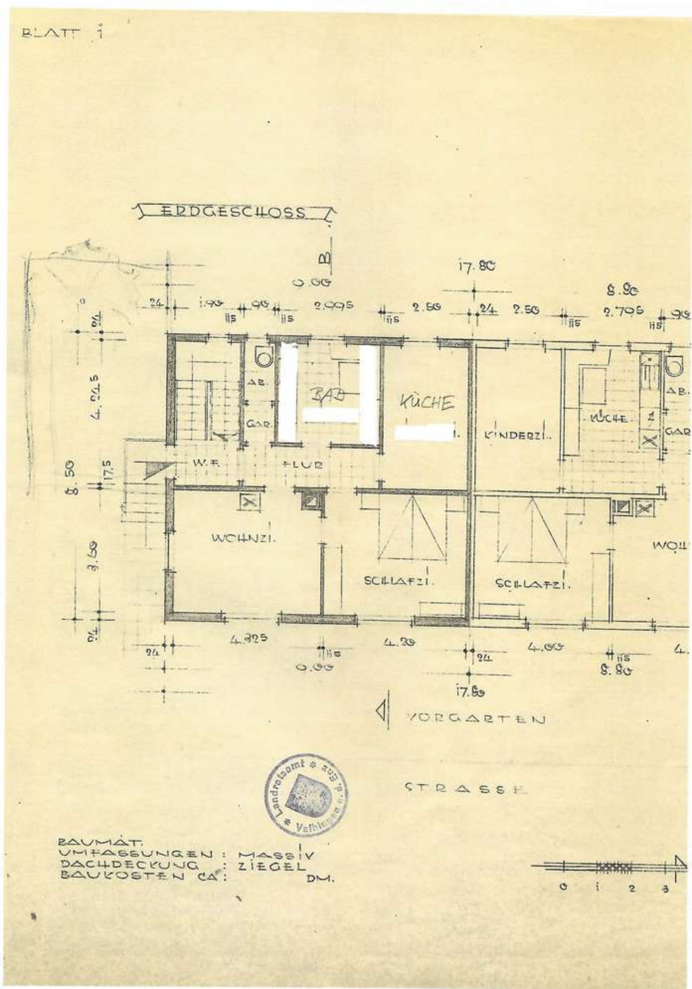
Grundriss_EG
