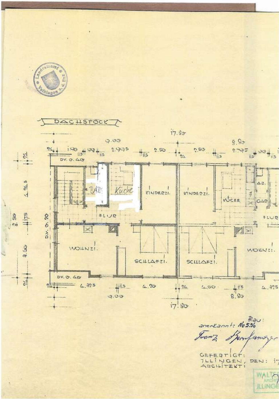
Grundriss_DG
